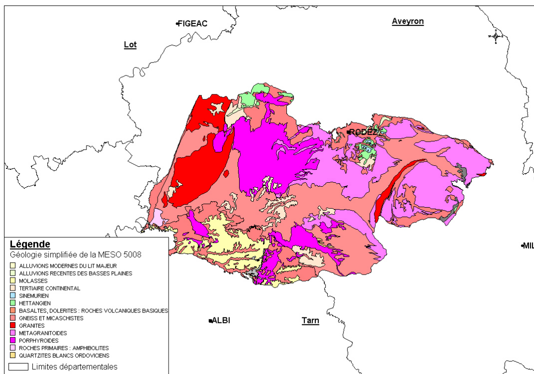
Géologie simplifiée de la masse d'eau 5008
